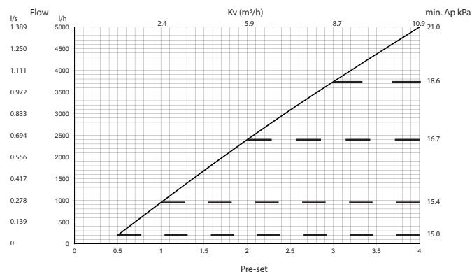
SIGMA Compact DN32
